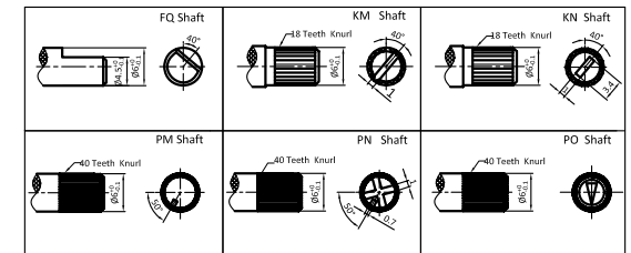
Shaft Options
