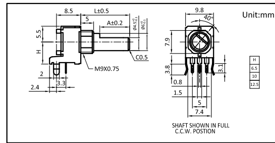
外型图
