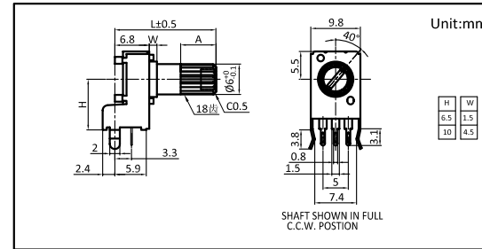
外型图
